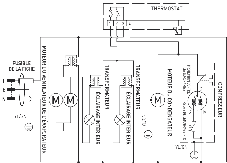
Schéma électrique (233931)
