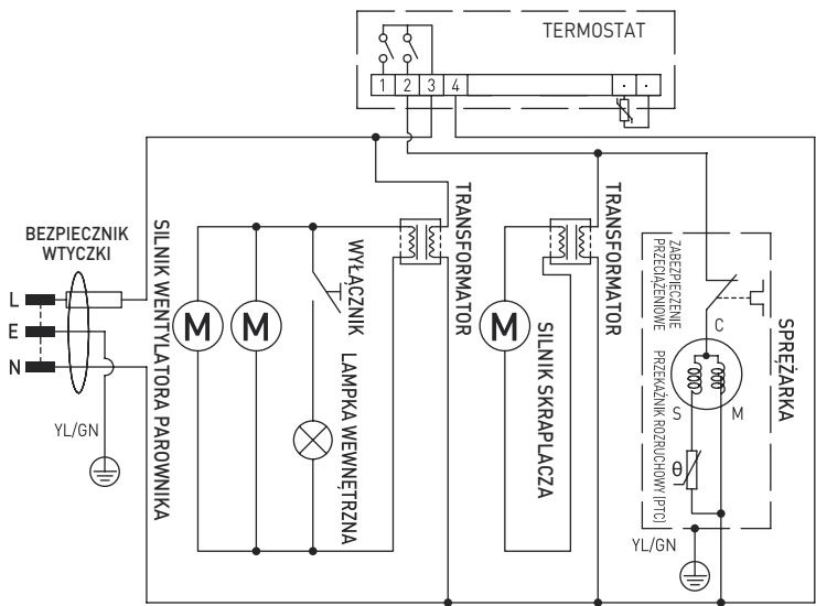
Schemat elektryczny (235836)
