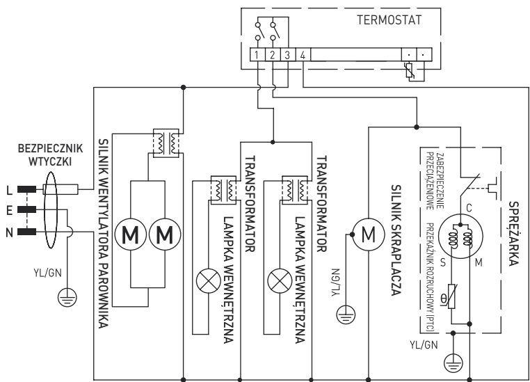
Schemat elektryczny (233931)
