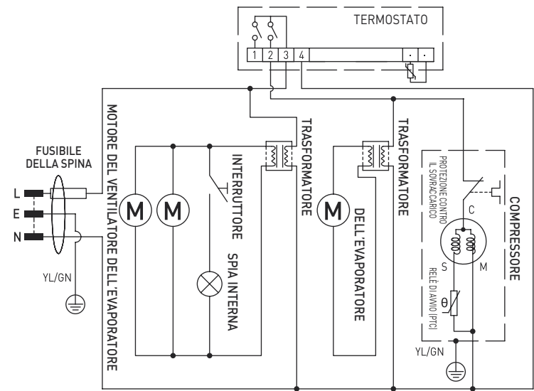
Schema elettrico (235836)
