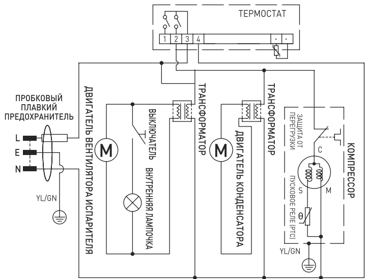
Электрическая схема (226568, 233900, 233917, 235829)
