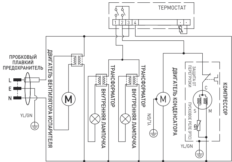
Электрическая схема (233924)
