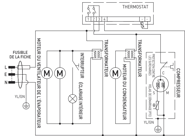
Schéma électrique (235836)
