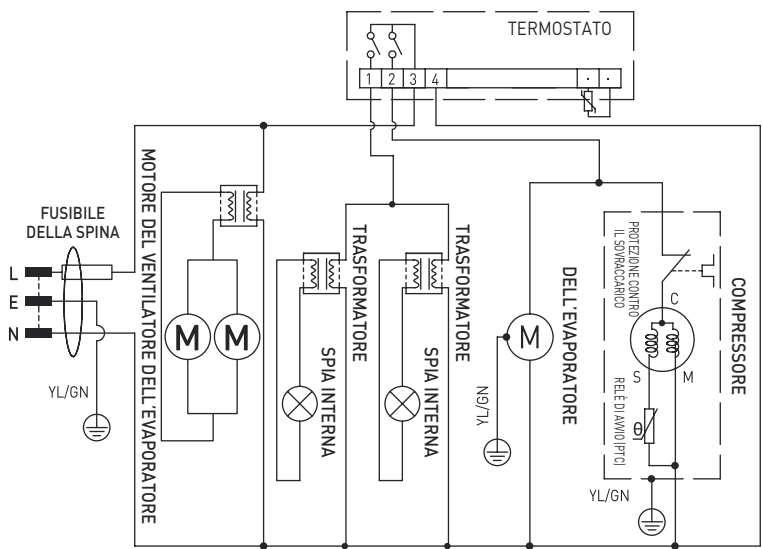
Schema elettrico (233931)
